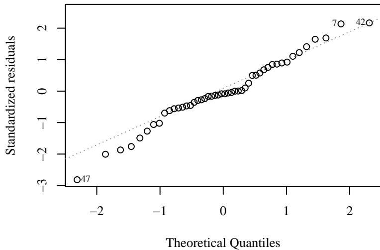
Normal Q-Q
