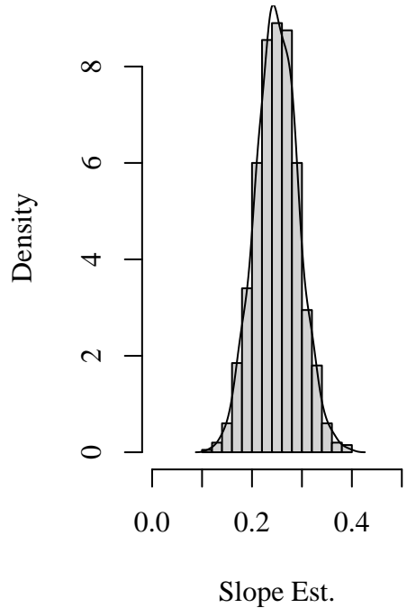
Homoskedastic Data
