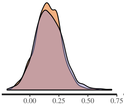
VoterXSent
