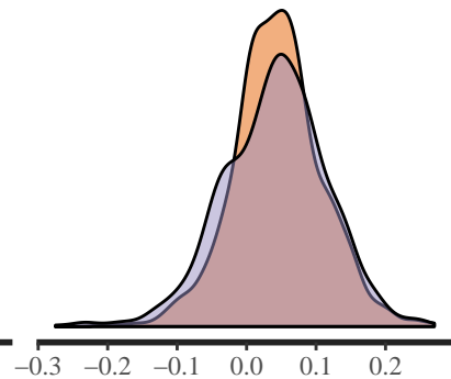
Voter^2
