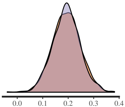
VoterXSent
