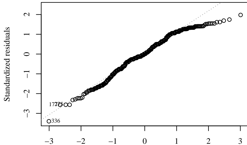
Normal Q-Q
