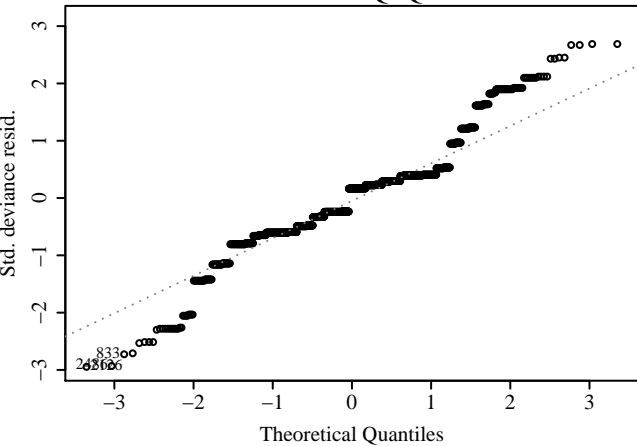
Normal Q-Q
