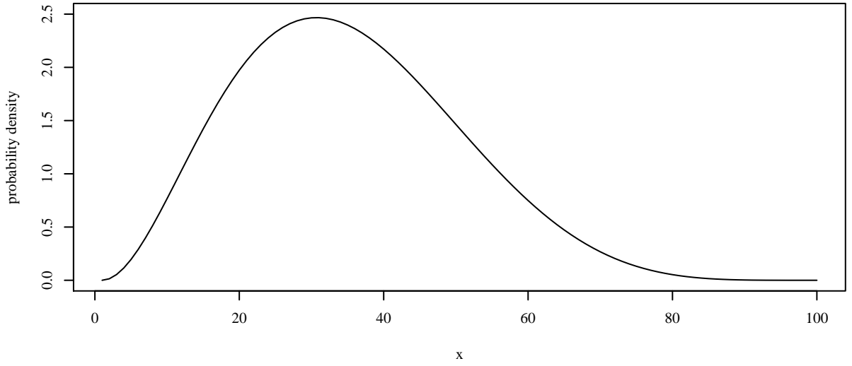
Beta( 3 , 5.67 )
