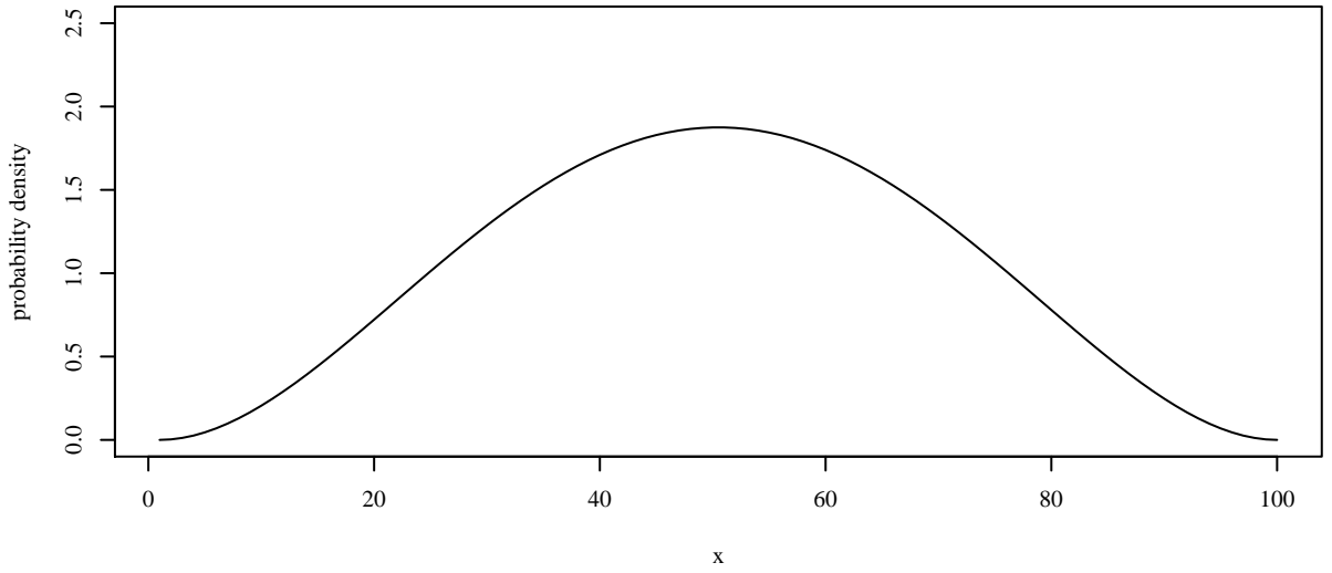
Beta( 3 , 3 )
