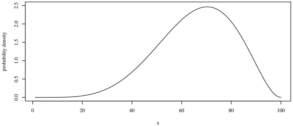
Beta( 5.67 , 3 )
